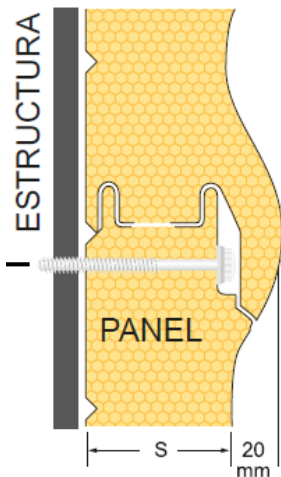
Detalle de la junta Longitudinal
